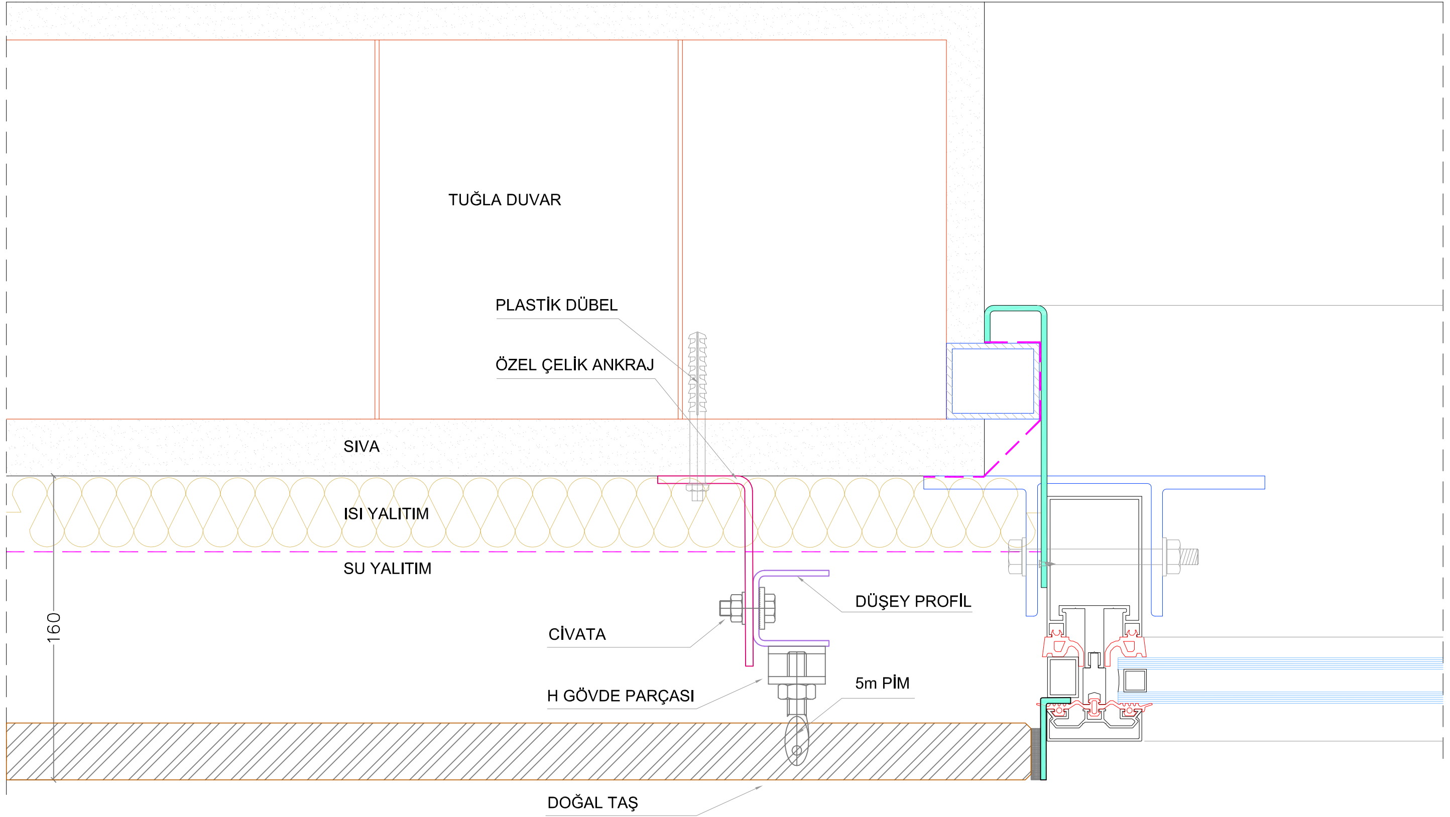
DETAY A
