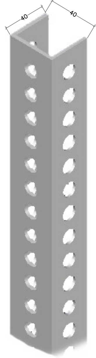
DÜŞEY PROFİL
