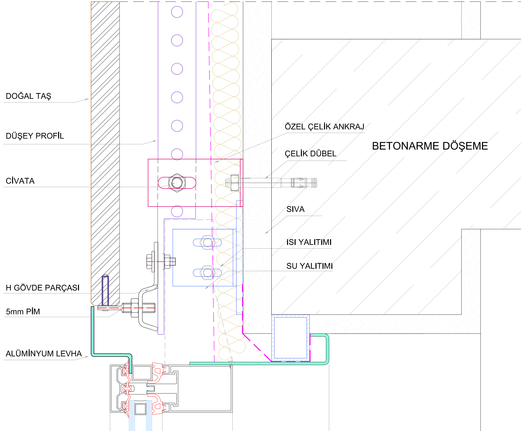
DETAY B
