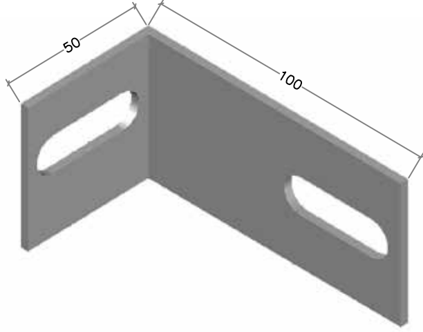
ÖZEL ÇELİK ANKRAJ
