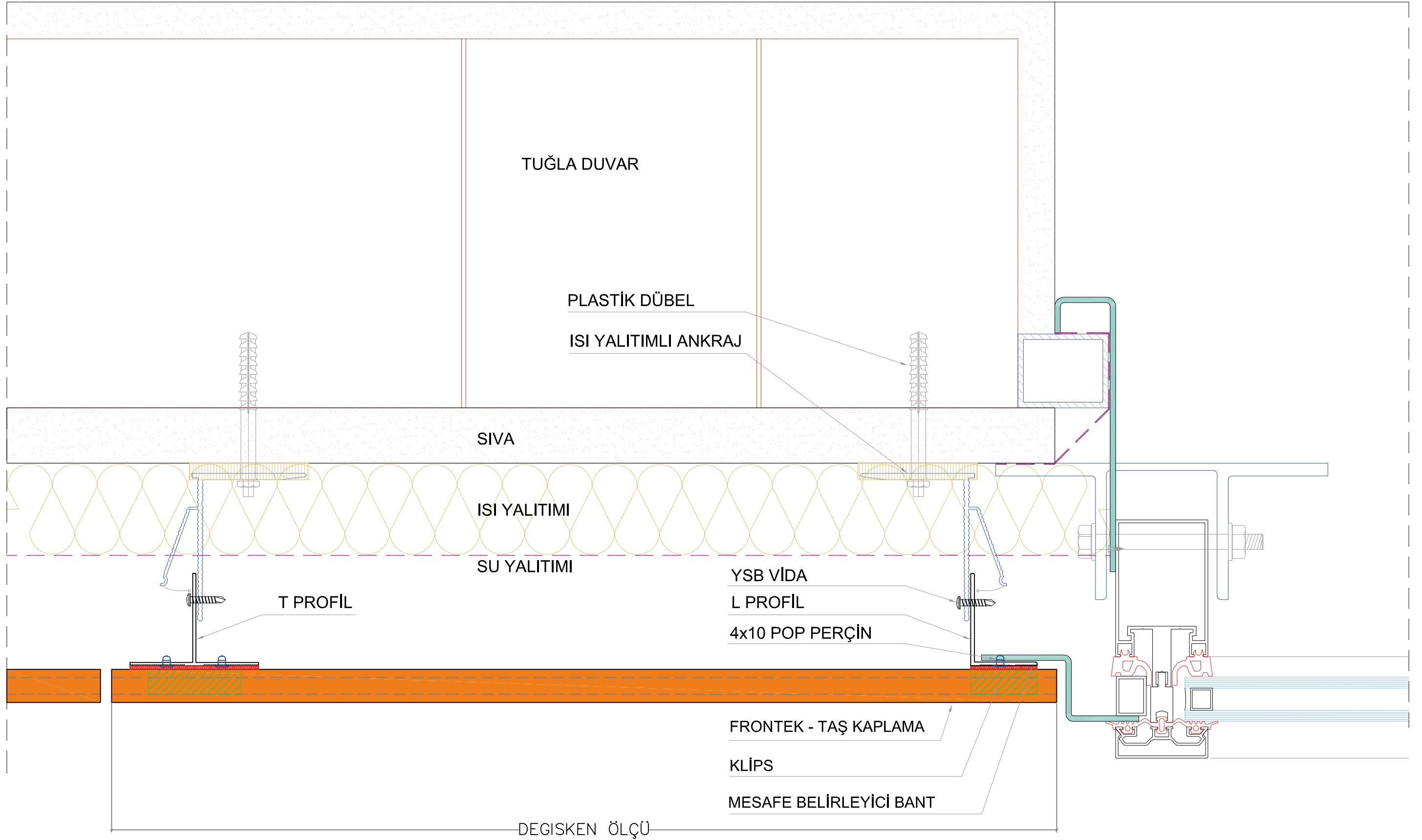
DETAY A
