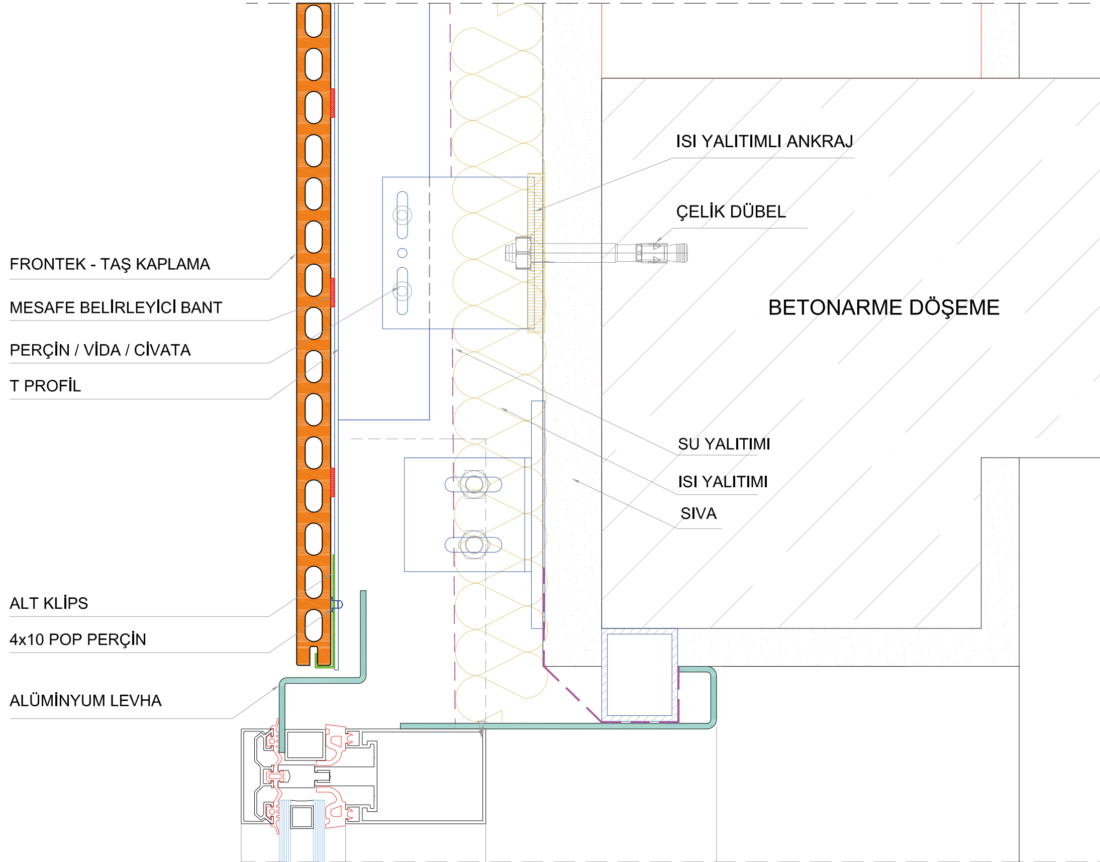
DETAY B
